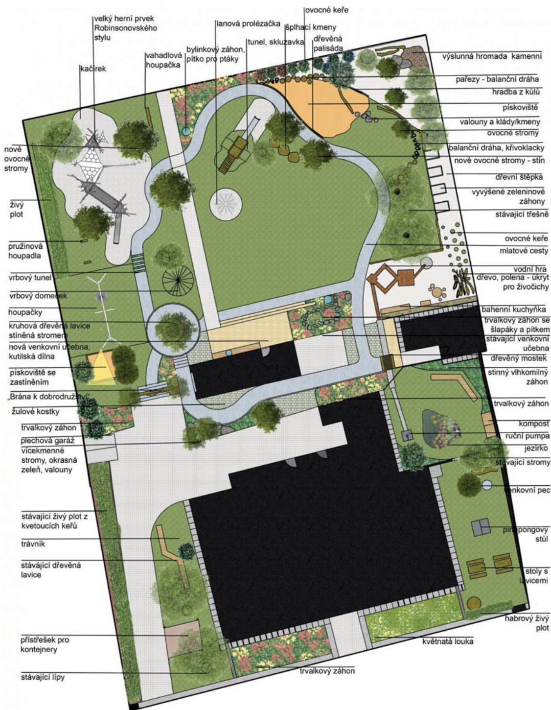
STUDIE ZAHRADY ZŠ A MŠ ŘEZNOVICE, K.Ú. ŘEZNOVICE. V/2023. SITUACE, FORMÁT VÝKRESU A3.
