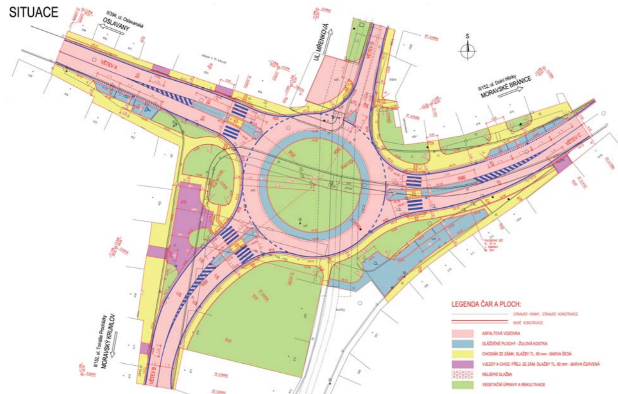
Obrázek 15 Situace - výkres plánované okružní křižovatky U Tří Kohoutů
